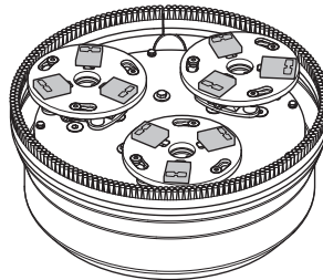
Volledige set - 3 Redi lock-schijfhouders, 9 schijven
